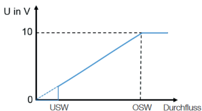
Spannungs-Durchfluss-Kennlinie
