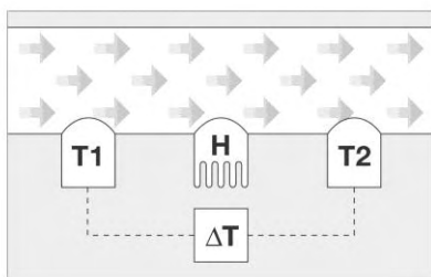
Abbildung 1: Messprinzip
