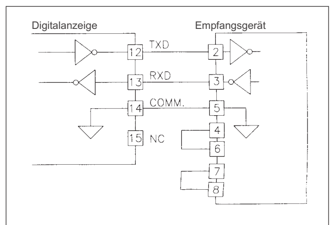
Bild VI: RS232-Schnittstelle
