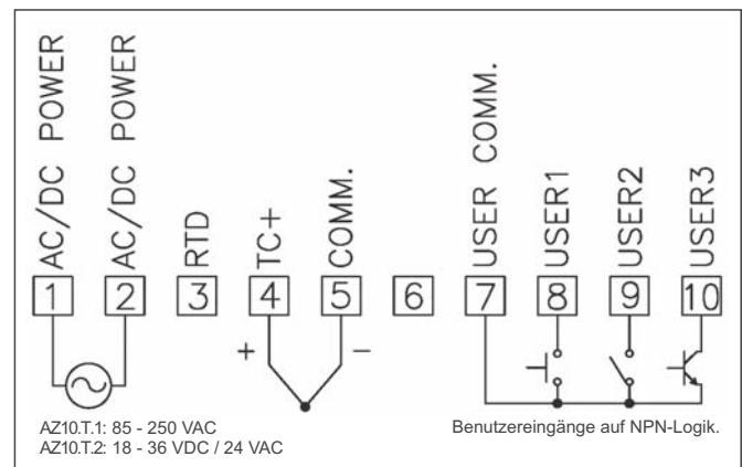
Bild 7.3: Anschluß eines Thermoelements
